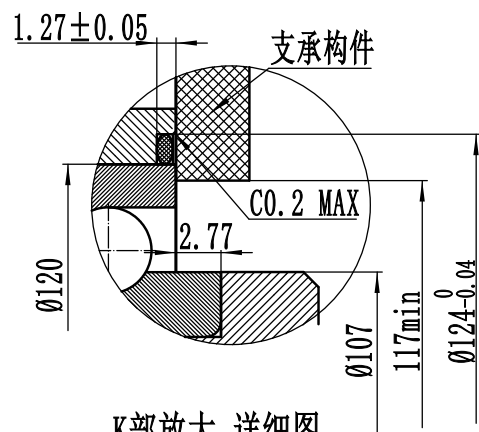
K部放大 详细图 4: 1
